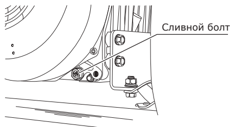
Рис. 18. Сливной болт
